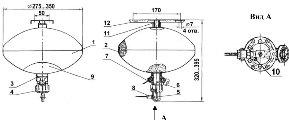
Рис. 1 Загальний вид модулів СПРУТ базових модифікацій «о» і «п»
