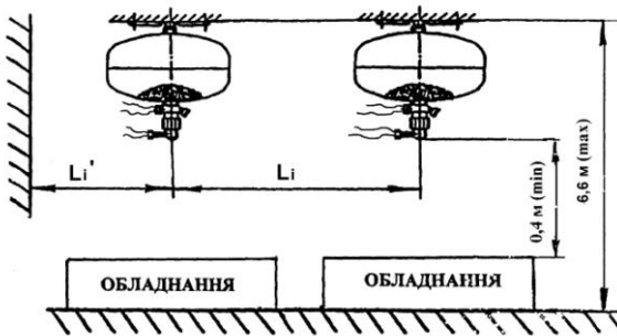
Рис. 3 Розташування модулів на захищаному об'єкті
